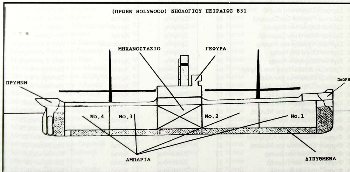
Πλάγια όψη της δεξιάς πλευράς του ατμοπλοίου «Τάναϊς» (πρώην Hollywood), νηολογίου Πειραιώς 831.
