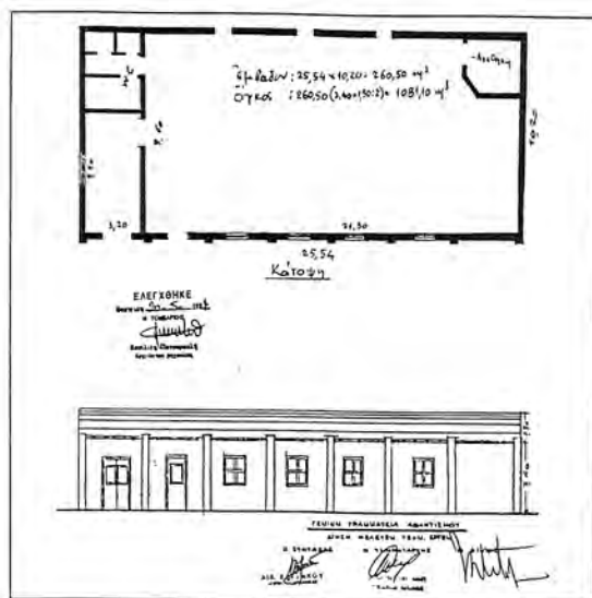
Εικ. 2: Σχέδιο του θαλάμου που στέγαζε τη Συναγωγή του συννοικισμού (Πολιτικός Αθλητικός Σύλλογος «Ναύαρχος Βότσης»).
